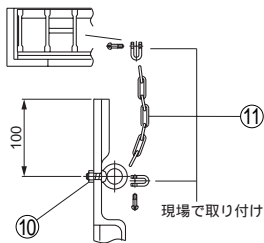
“a”部詳細 S=1:2
