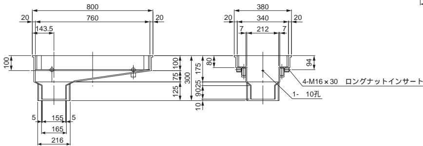
“a”部詳細 S=1:2
